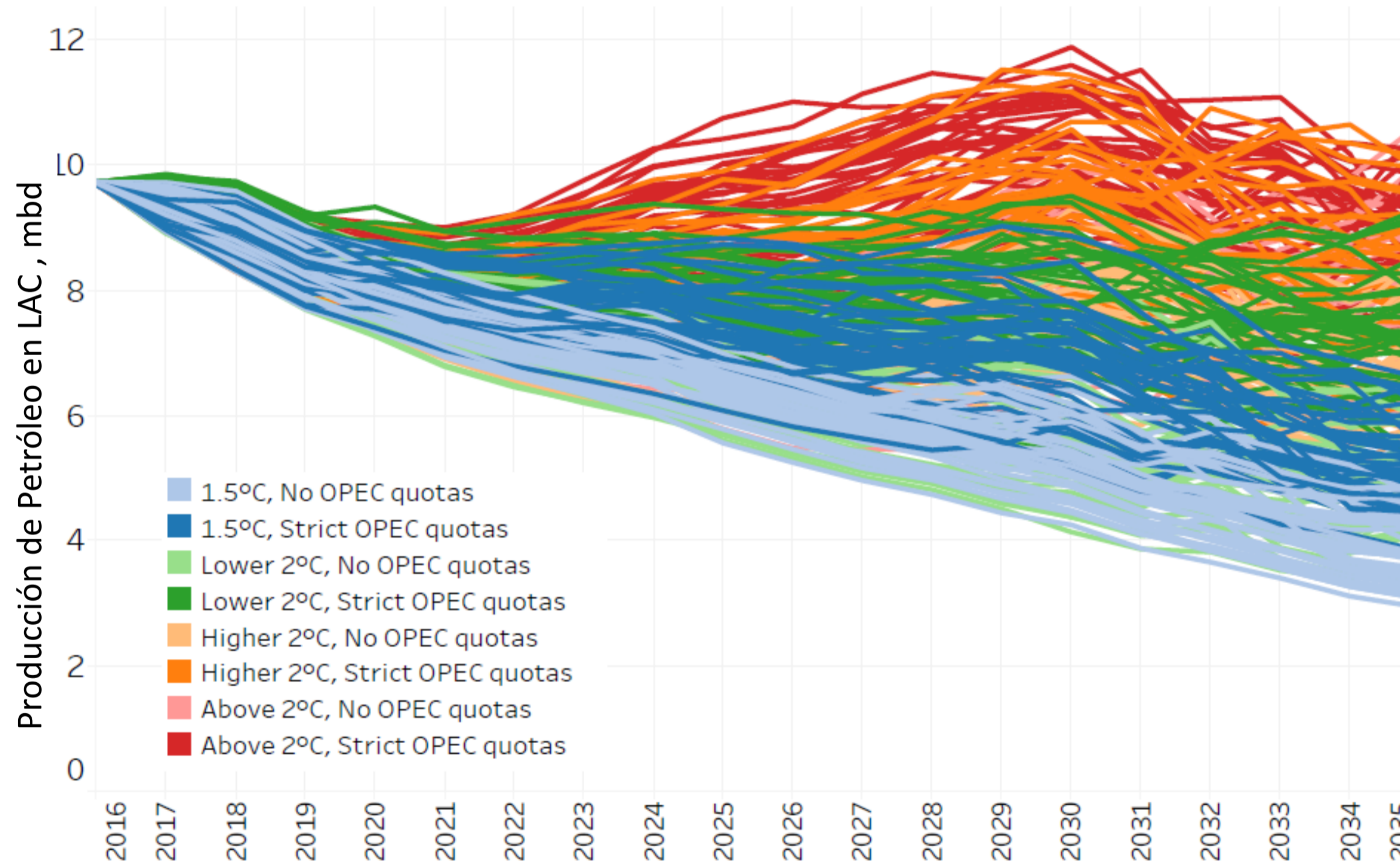
Escenario de producción de Petróleo en LAC según cambio global en temperatura
